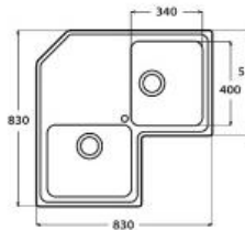
Horní montáž
