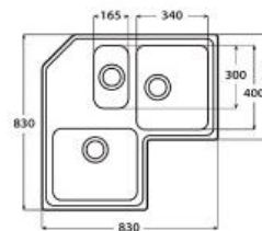
Spodní montáž
