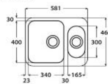
Spodní montáž
